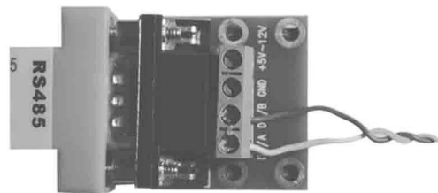
(شکل شماره ۲ نمونه پورت RS232/RS485 با تغذیه 5VDC)
