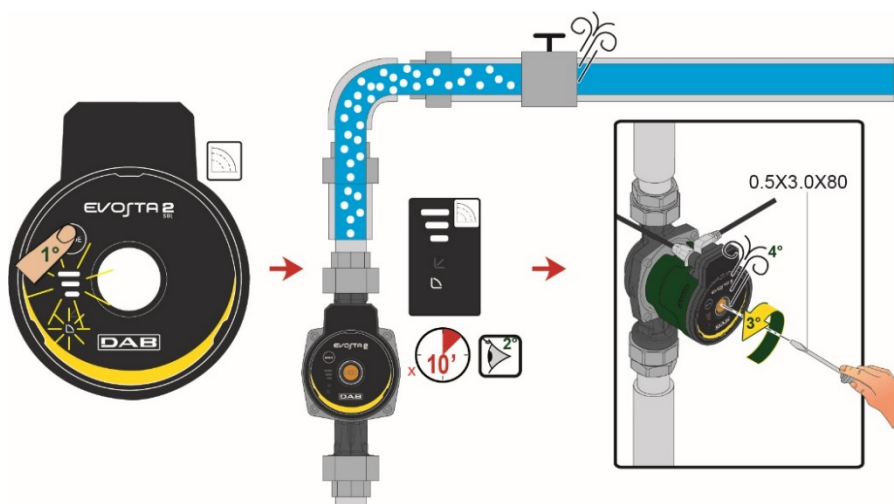
Slika 17: Odzračitev črpalke
