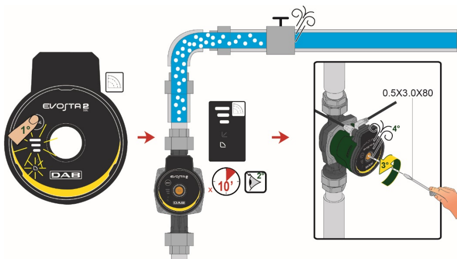
Figura 17: Aerisirea pompei
