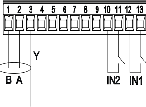
Resim 7: 13 kutuplu çekmeceli klemens kutusu: Dijital girişler ve MODBUS
