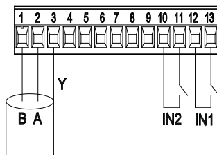
Obr. 7: Vyberateľná 13-pólová svorkovnica: digitálne vstupy a MODBUS
