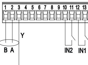
7 pav. Ištraukiama 13 kontaktų gnybtų dėžutė skaitmeniniams įvadams ir MODBUS
