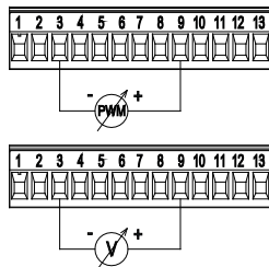
Figura 8: Morsettieria estraibile 13 poli: ingressi 0-10V e PWM
