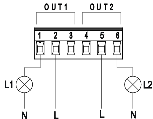
9 pav. Ištraukiama 6 kontaktų gnybtų dėžutė. Išvadu sujungimo pavyzdys
