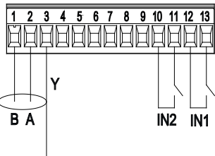
Kuv. 7: 13-napainen ulosvedettävä riviliitin: digitaaliset tulot ja MODBUS
