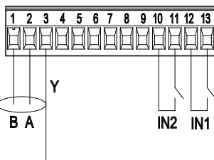
7. ábra: 13 pólusú kivehető sorkapocs tábla: Digitális bemenetek és MODBUS
