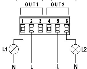
Figura 9: Morsettieria estraibile 6 poli: esempio di collegamento uscite
