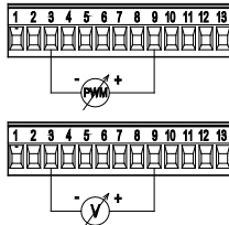
Εικόνα 8: Αφαιρούμενη κλέμμα 13 πόλων: είσοδοι 0-10V και PWM
