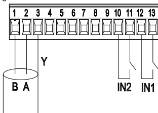
Afbeelding 7: Uittrekbaar 13-polig klemmenbord: digitale ingangen en MODBUS
