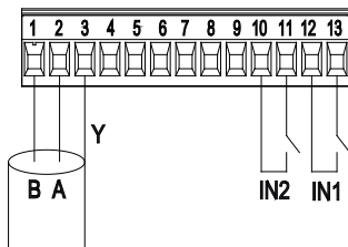
Εικόνα 7: Αφαιρούμενη κλέμμα 13 πόλων: ψηφιακές εισοδοι και MODBUS
