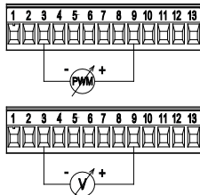
Abbildung 8: Abnehmbares Klemmenbrett mit 13 Polen: Eingänge 0-10V und PWM
