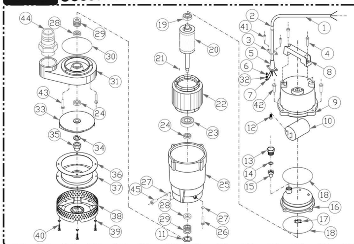
لیست قطعات استفاده شده در پمپ لجن کش SI-25-1
