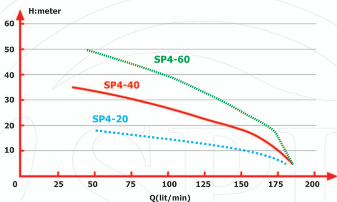
منحنی میزان آبدهی - ارتفاع
